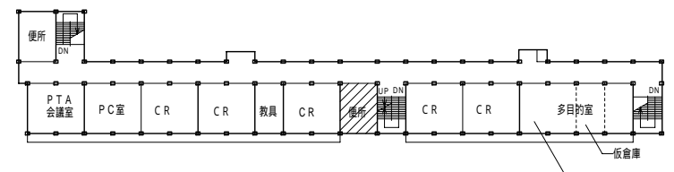
4階 平面図 1/500
