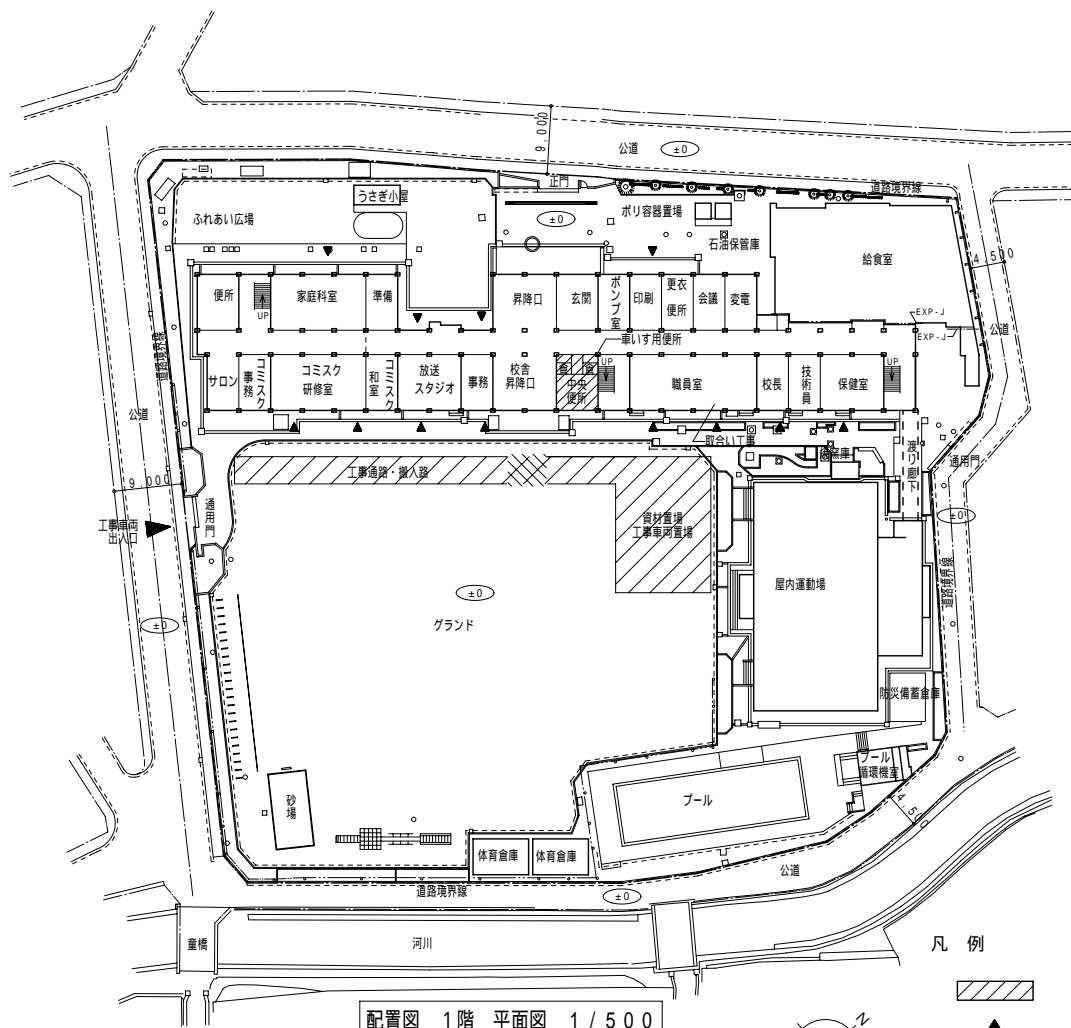
配置図 1階 平面図 1/500
